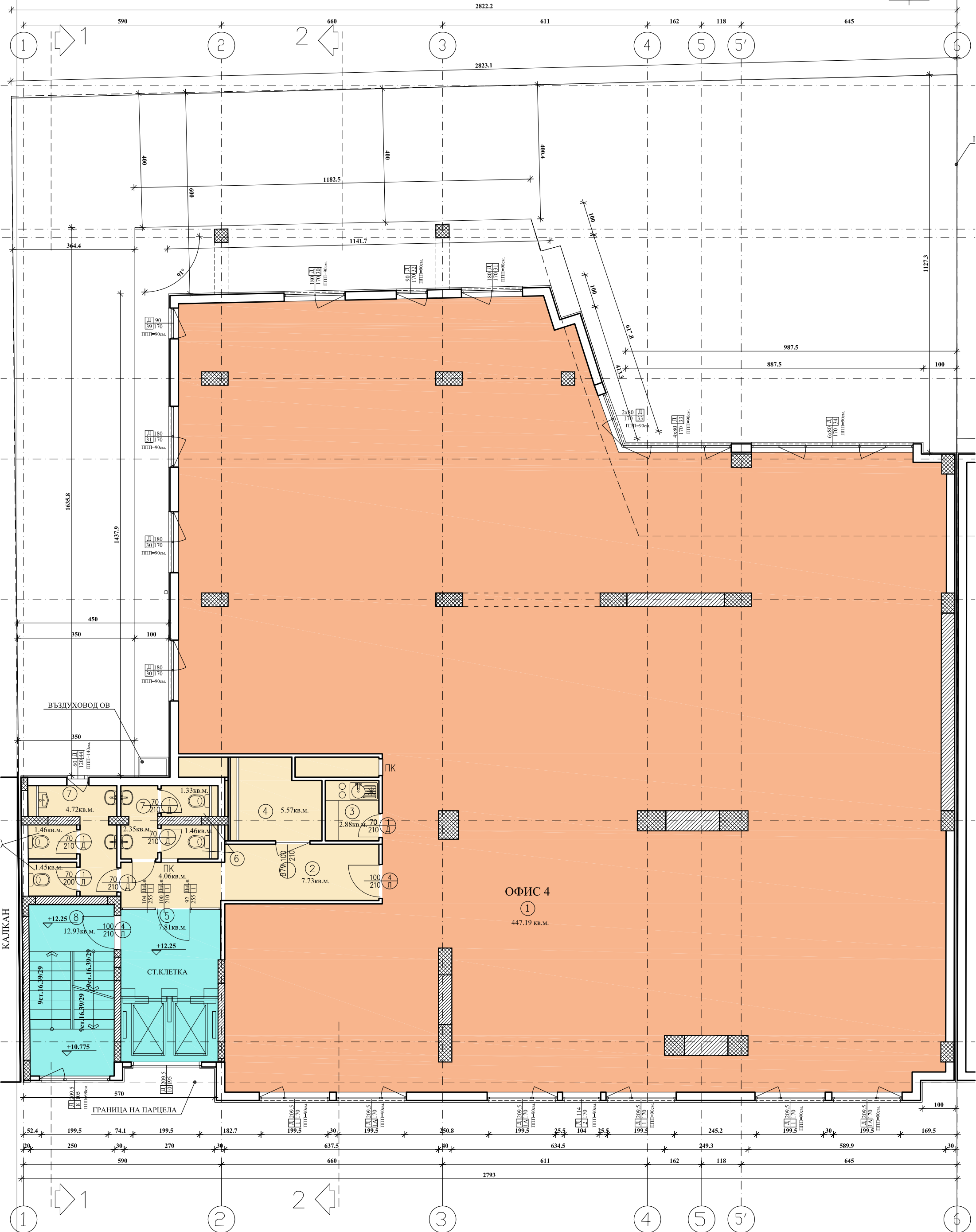
РАЗПРЕДЕЛЕНИЕ 4 ЕТАЖ М 1:100 Площ = 558.11 м 2
