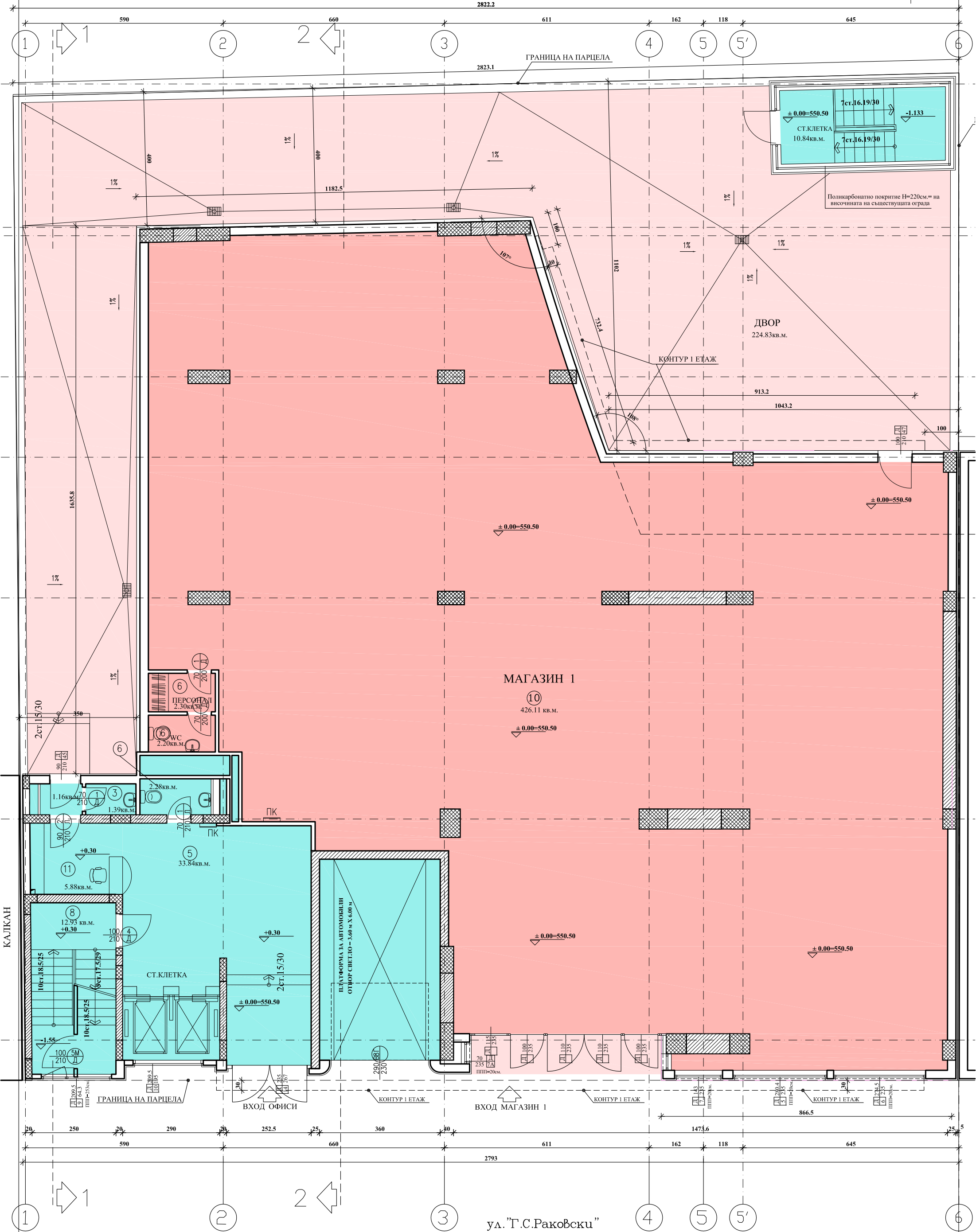
РАЗПРЕДЕЛЕНИЕ ПАРТЕРЕН ЕТАЖ М 1:100 Площ = 834.32 м 2
