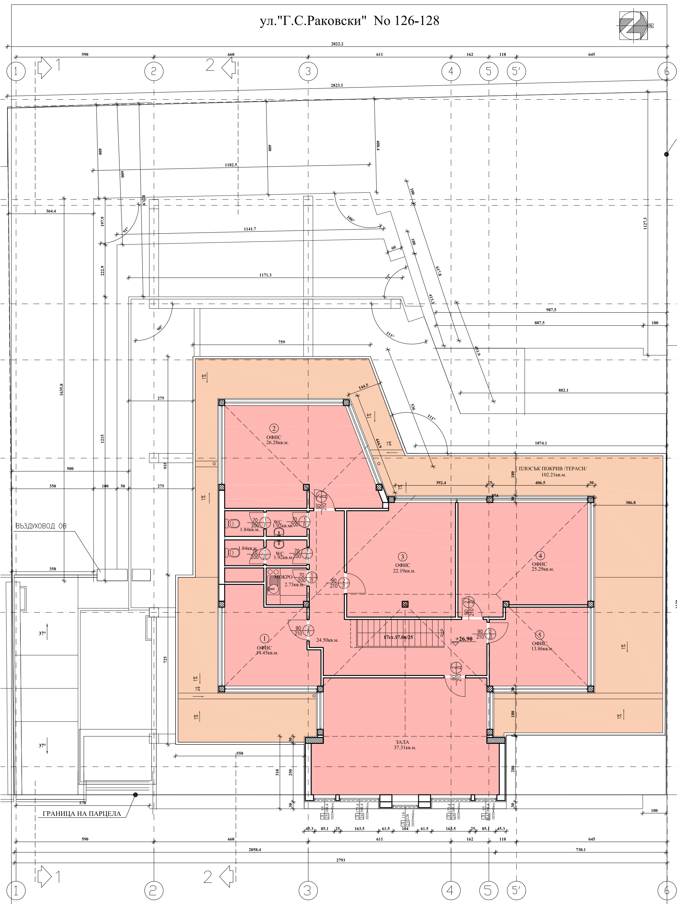
РАЗПРЕДЕЛЕНИЕ КОТА +26.90 М 1:100 Площ = 313.38 м 2
