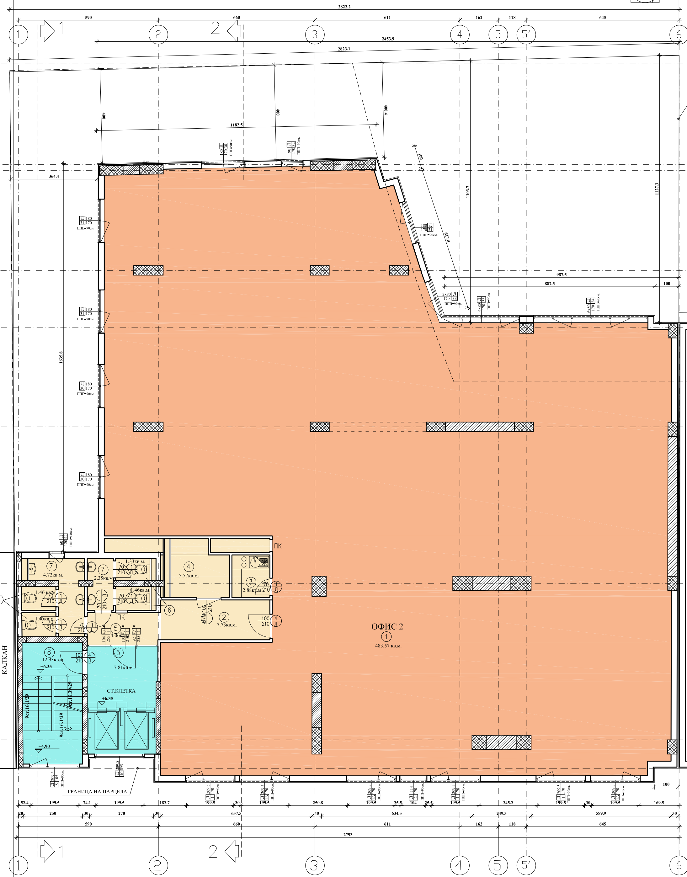
РАЗРЕДЕЛЕНИЕ 2 ЕТАЖ М 1:100 Площ = 598.01 м 2
