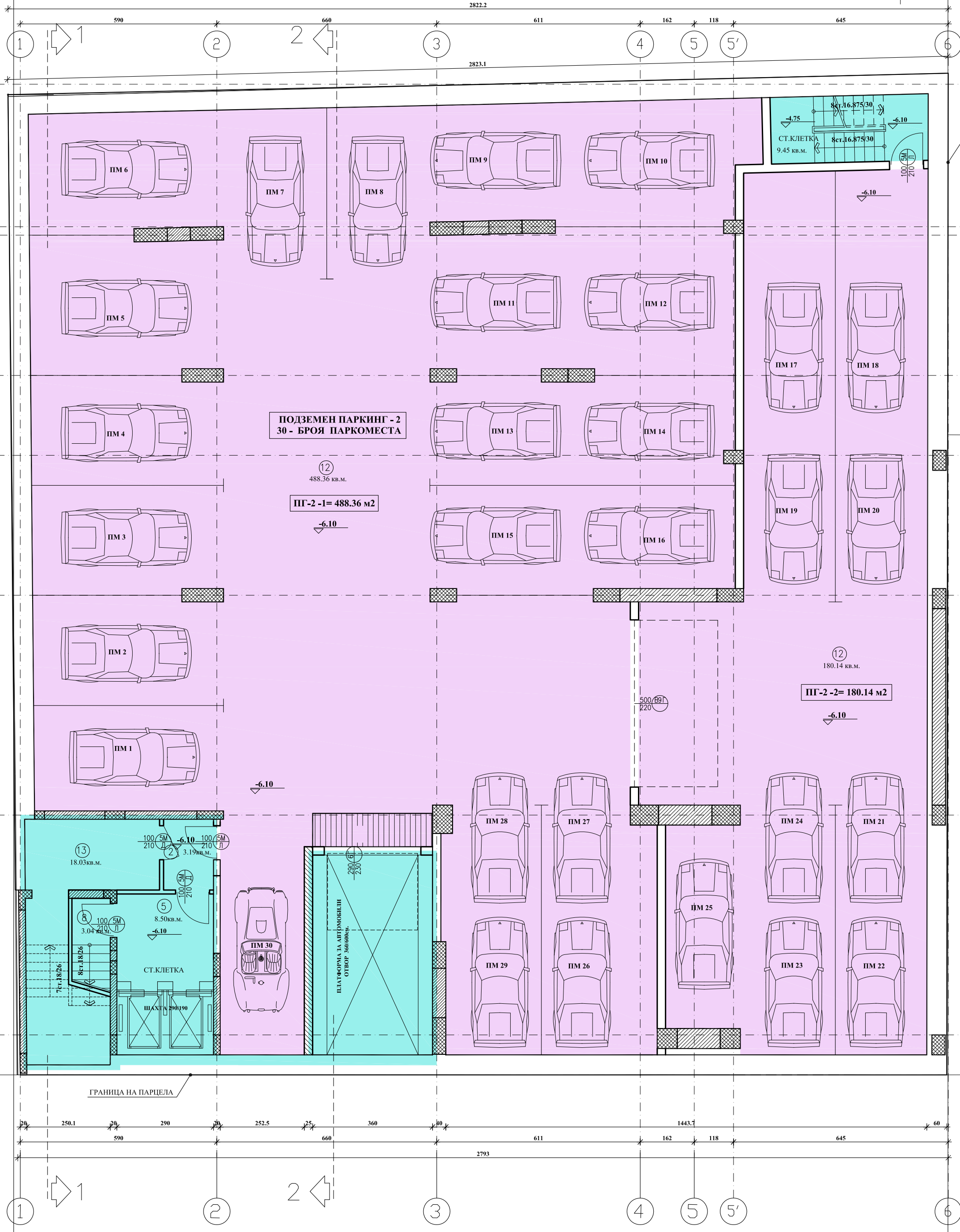
РАЗПРЕДЕЛЕНИЕ 2 СУТЕРЕНЕН ЕТАЖ М 1:100 Площ = 834.32 м2
