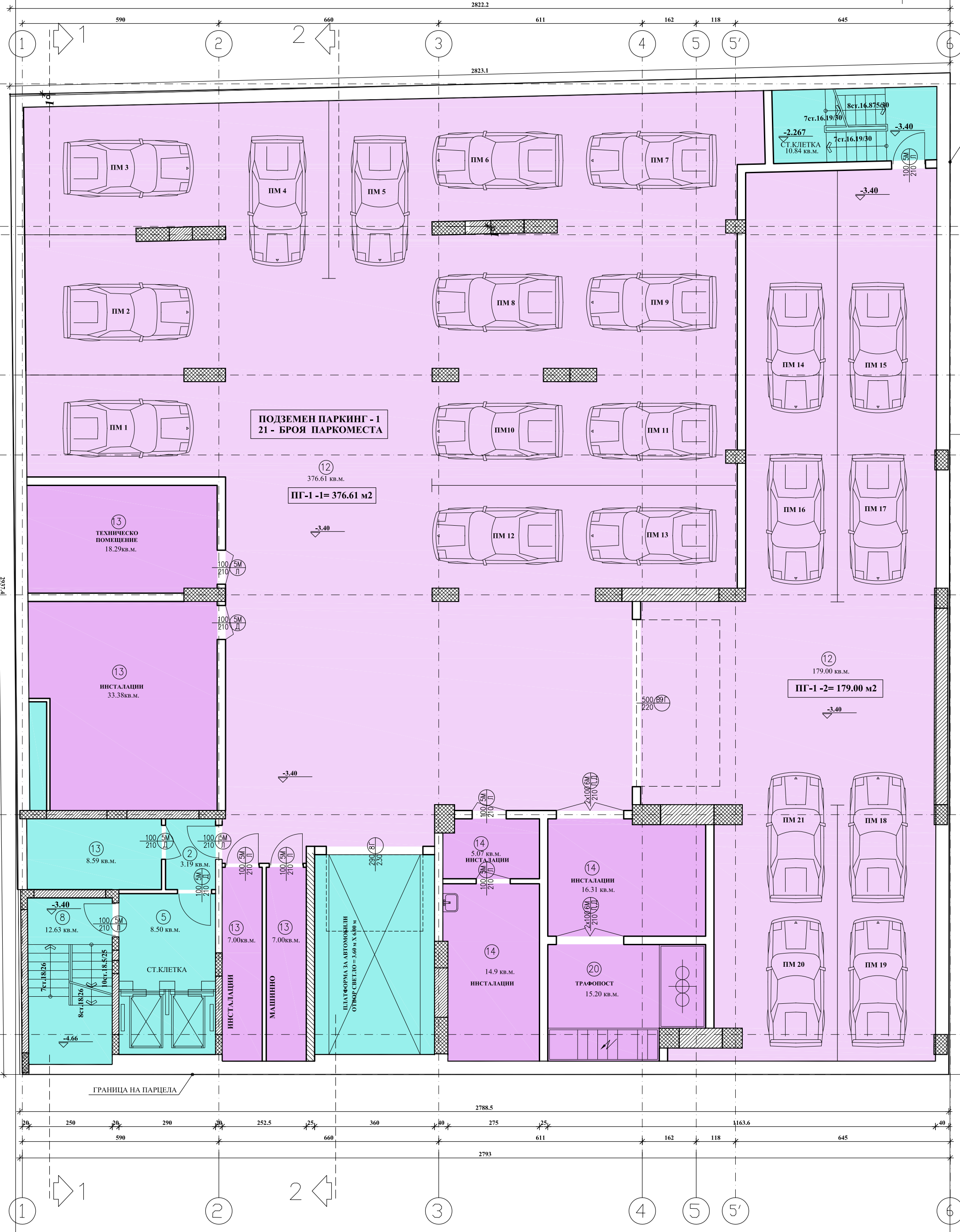
РАЗПРЕДЕЛЕНИЕ 1 СУТЕРЕНЕН ЕТАЖ М 1:100 Площ = 834.32 м 2
